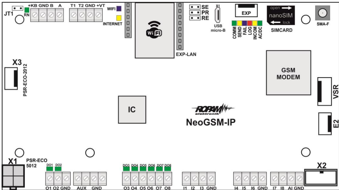
Widok: NeoGSM-IP PCB.
