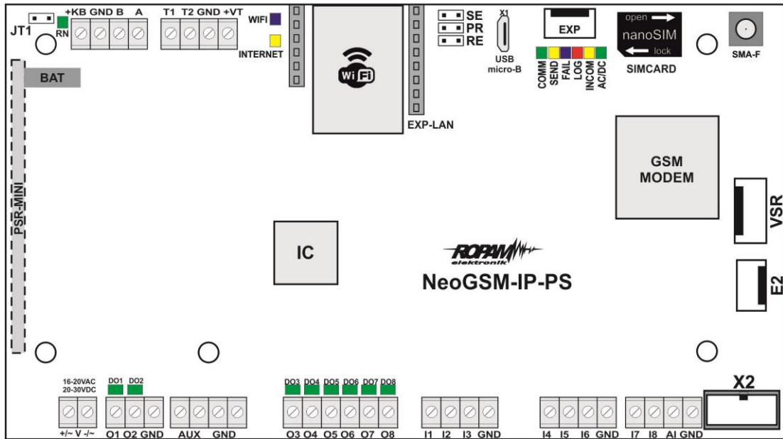
Widok: NeoGSM-IP-PS PCB.
