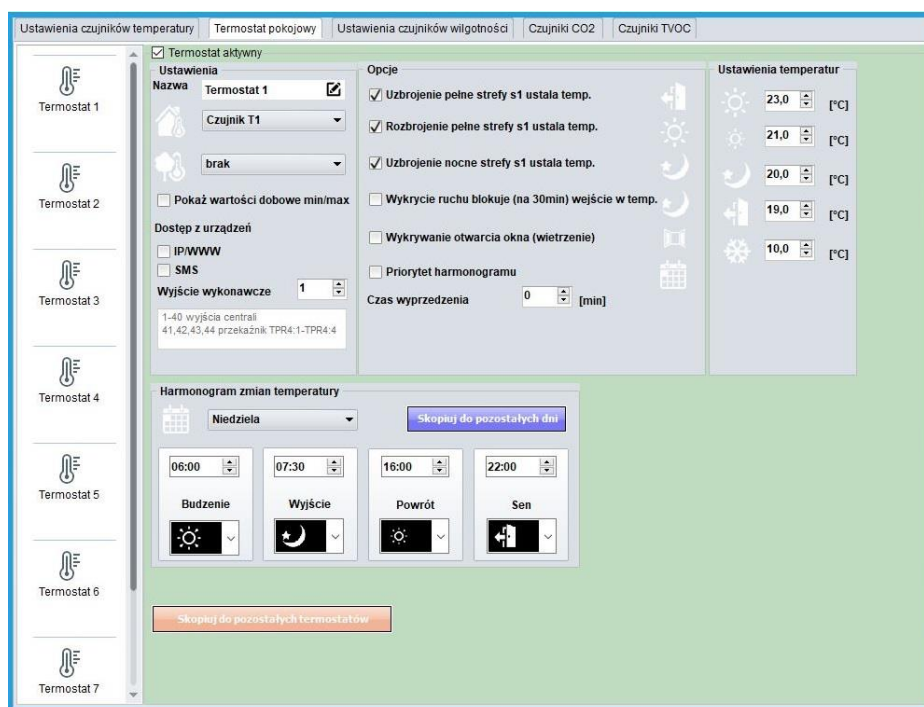
Okno ustawień termostatów – NeoGSMIP64 Manager:
