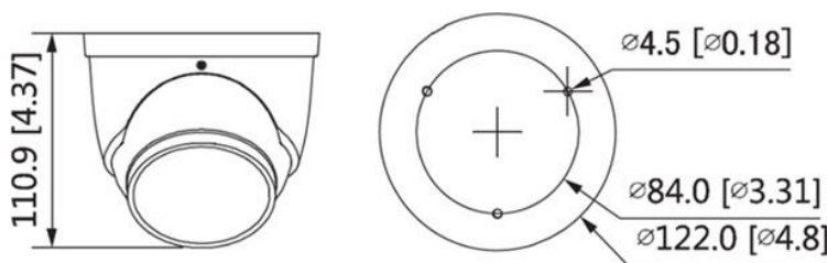
Ilustracja 3-1 Wymiary (jednostka: mm [cale])
