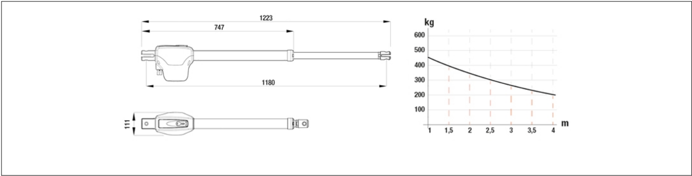
WYMIARY
