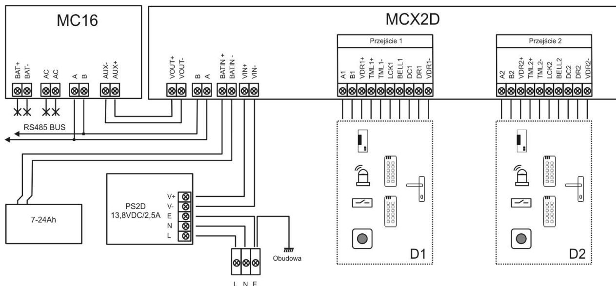
Rys. 6 Schemat połączeń pomiędzy ekspanderem i kontrolerem zasilanym z ekspandera
