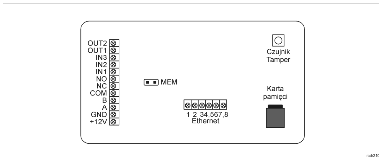
Rys. 7 Wewnętrzna strona panelu przedniego
