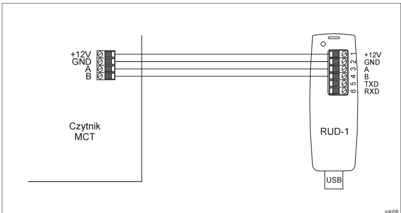
Rys. 10 Sposób podłączenia terminala do interfejsu RUD-1.
