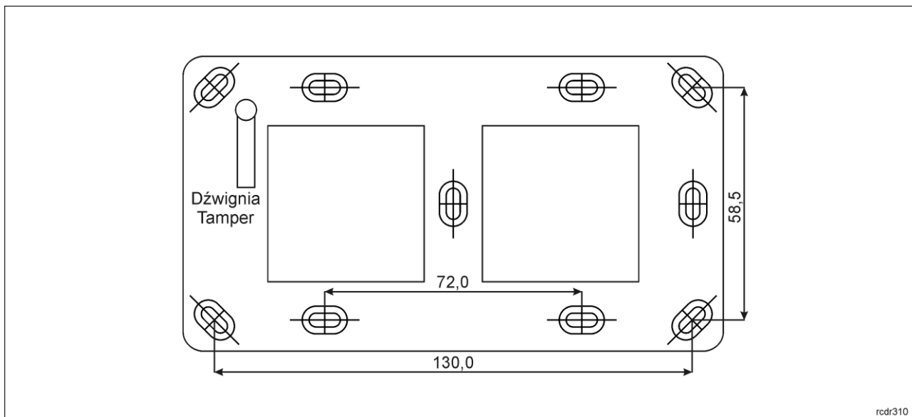
Rys. 8 Panel tylny
