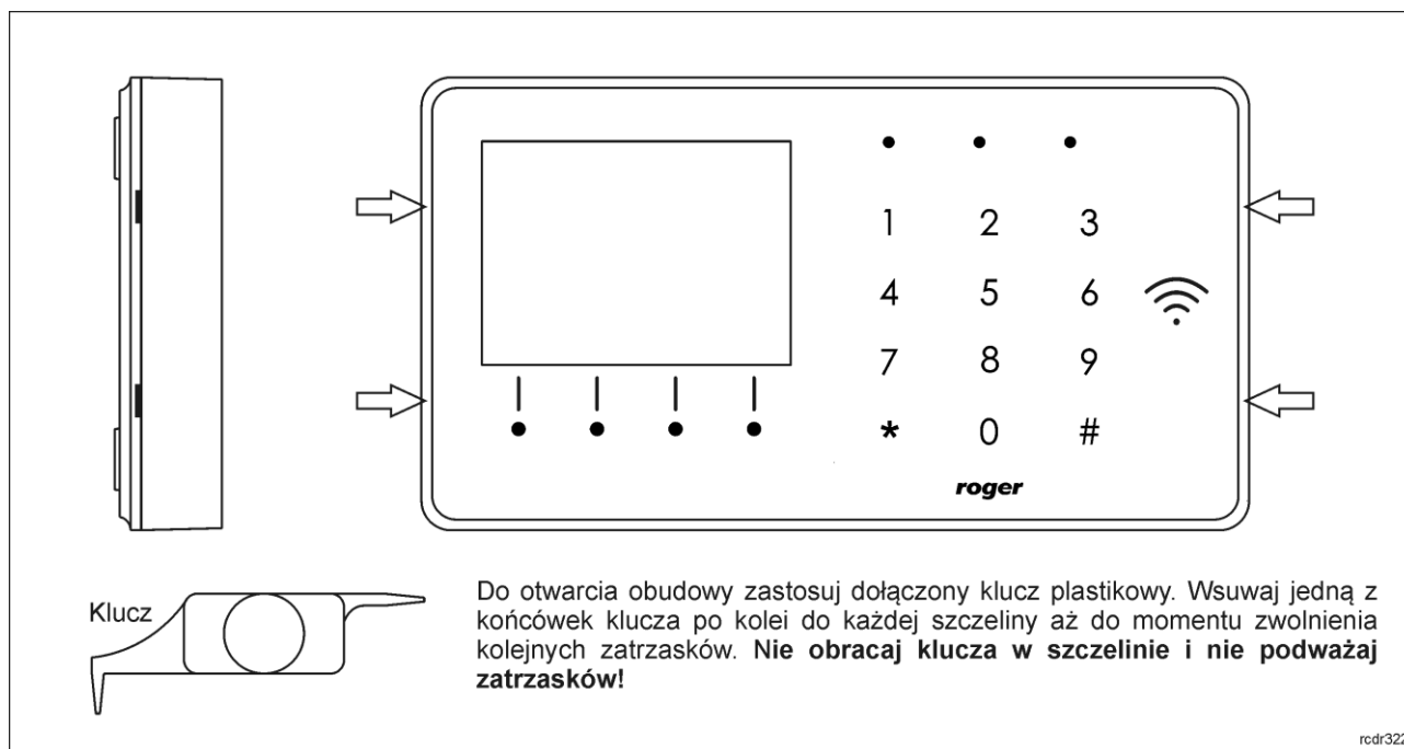
Rys. 6 Demontaż obudowy urządzenia
