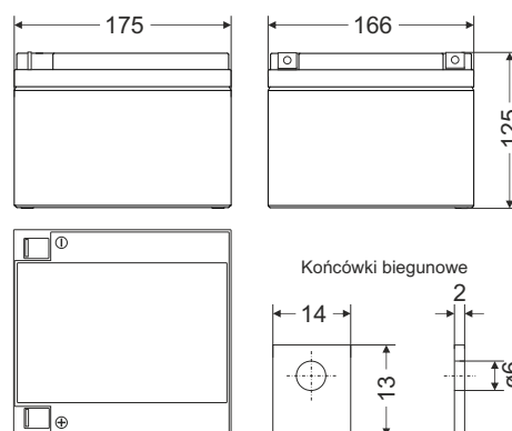
Wymiary w [mm] Tolerancja: +/- 2mm;
