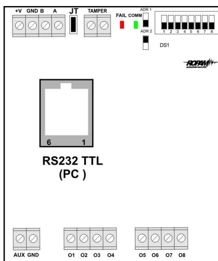
Widok modułu EXP-I8-RN
