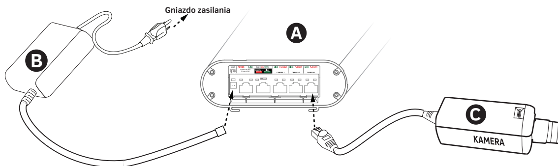
Rys. 2 Schemat podłączenia urządzeń według opcji 1
