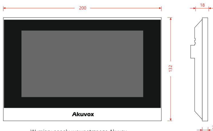
Wymiary panelu wewnętrznego Akuvox
