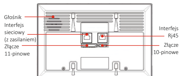
Złącza panelu Akuvox
