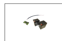
BI/BAT/KIT Kit zestaw do awaryjnej adowarki akumulatorów do sterownika cyfrowego Brushless CTRL 36V DC w komplecie z 2 bateriami 12V DC 4,5 Ah. Zestaw szlabany BIONIK.
