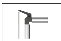
SND/BA/68/UP/RD cznik z przegubem 90° z drkiem górnym (wersja obniona) do prt BA/68.
